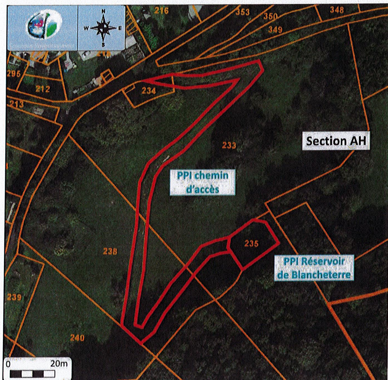
ANNEXE 3 : plan du périmètre de protection immédiate du réservoir et du chemin d'accès
