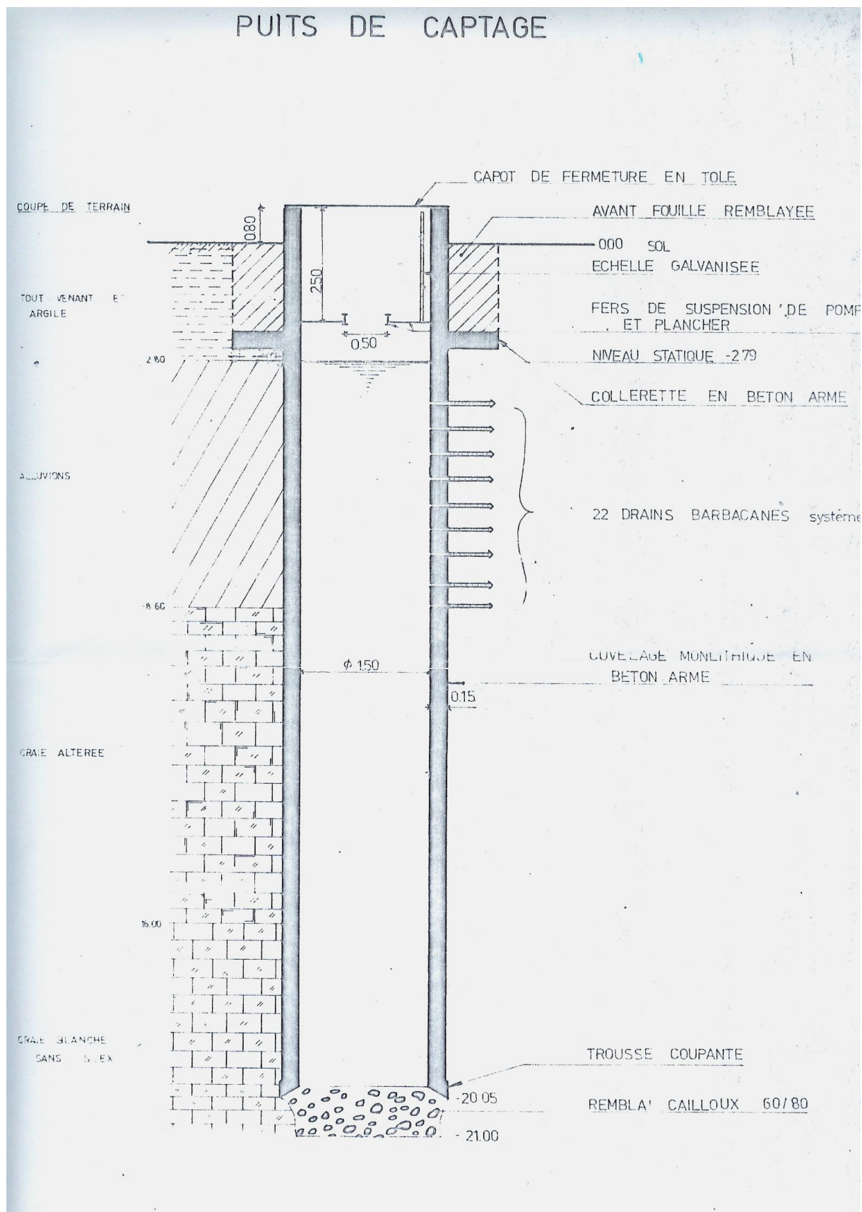
Figure 03 : Coupe technique du puits d'Entre-deux-Noues (confirmée par l'inspection vidéo Tauw)
