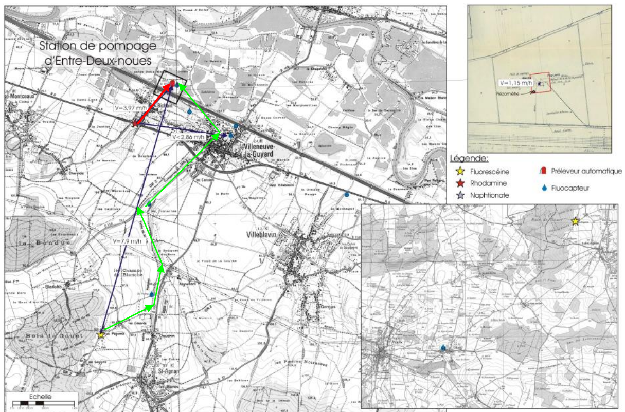
Figure 07 : Résultats des traçages (extrait Sciences-Environnement)
