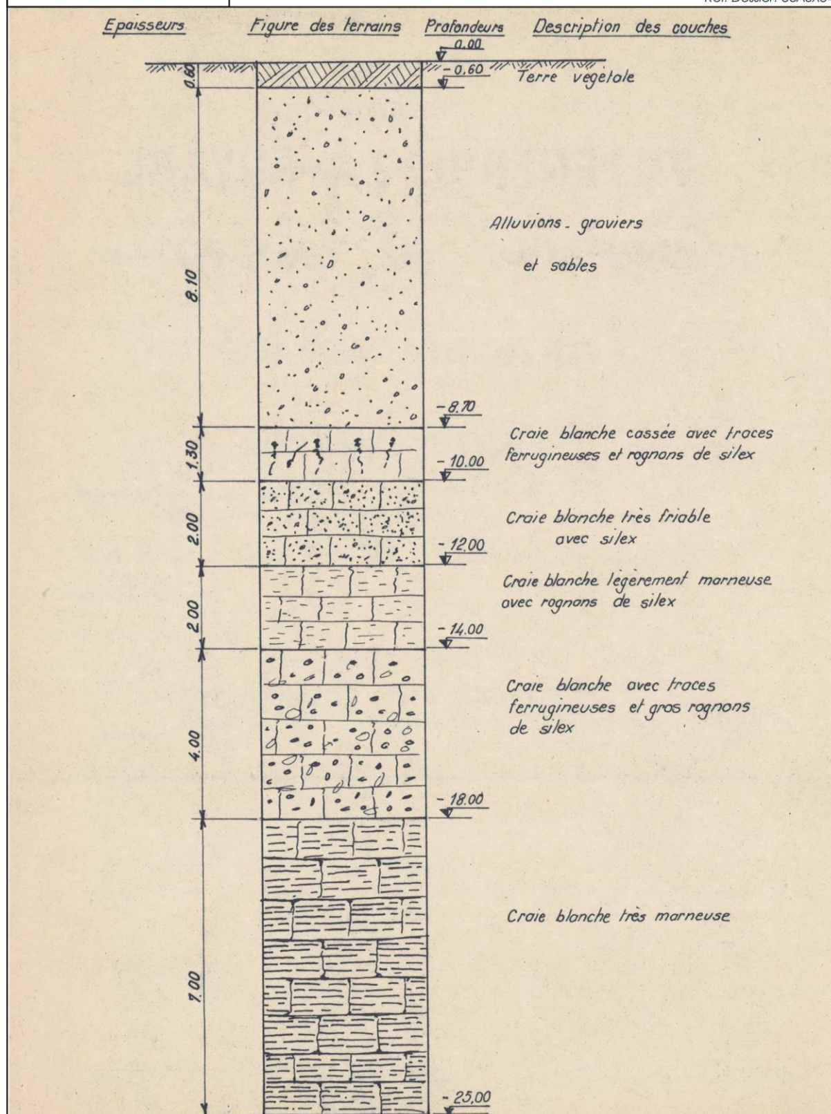
Fig. 3: Coupe lithologique de sondage du puits d'Entre-Deux-Noues
