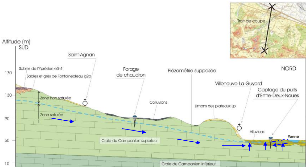
Figure 05 : Coupe géologique (extrait dossier de déclaration STEP de Saint-Agnan - Sciences Environnement)
