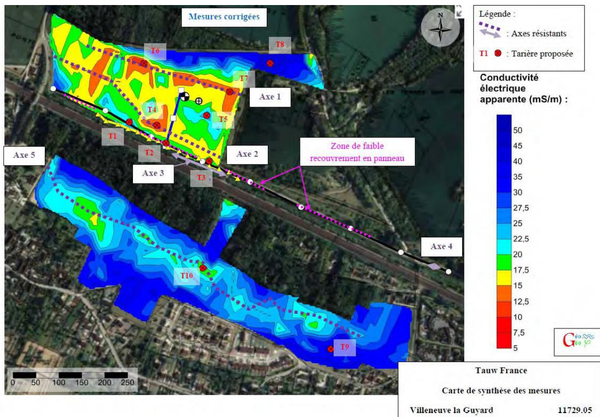
Figure 09 : résultats de la prospection géophysique
