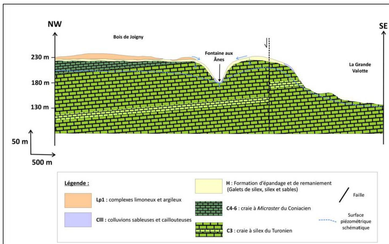
Figure 5 : contexte géologique (extrait rapports Sciences Environnement)
