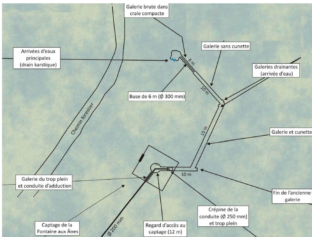
Figure 4 : Schéma de la galerie de captage (selon Sciences Environnement)
