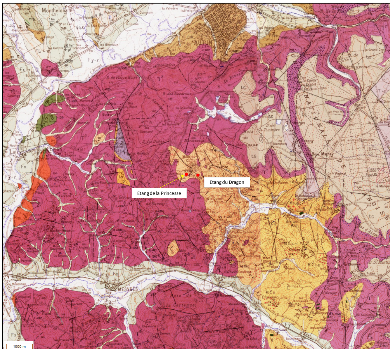
Figure 14 : localisation de l'étang du Dragon et de l'étang de la Princesse sur extrait de carte géologique au 1/50 000° d'AUTUN
