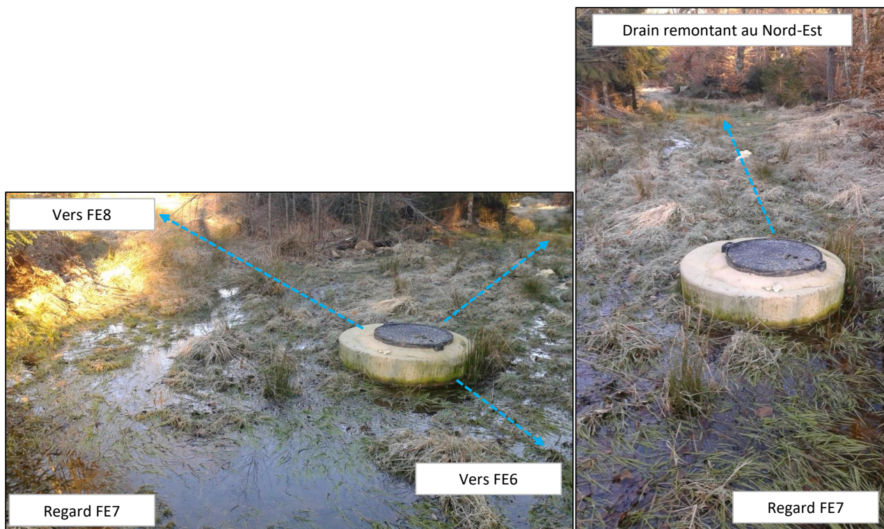
Figure 12 : le regard FE7 et ses ramifications
