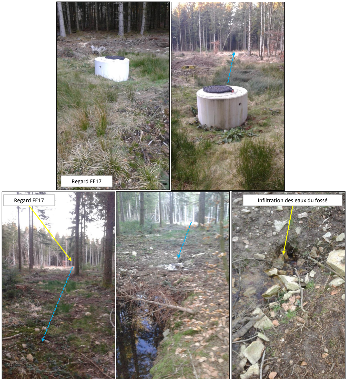
Figure 8 : le regard de La Fée amont : l'ouvrage FE17 et le drain de 130 m en direction de la zone boisée avec infiltration des eaux du fossé juste en amont du drain repris
