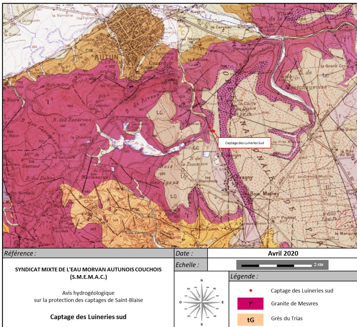
Figure 4 : localisation du captage des Luineries sud sur extrait de carte géologique au 1/50 000 e , feuille d'Autun
