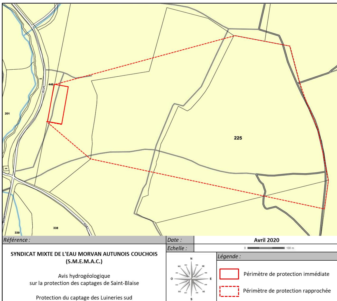
Figure 9 : délimitation du périmètre de protection rapprochée du captage des Luineries sud sur fonds IGN et cadastral
