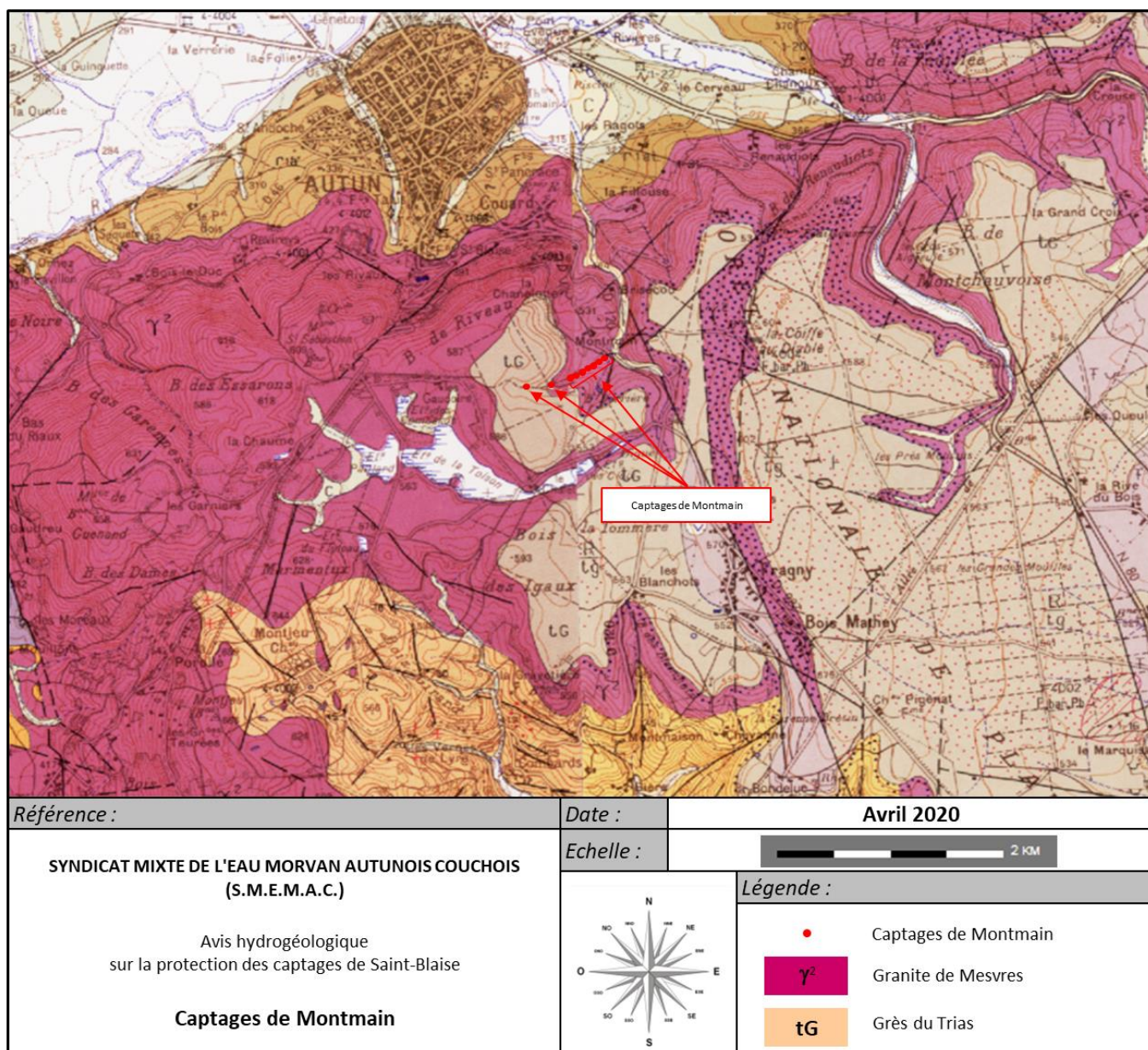
Figure 4 : localisation des captages de Montmain sur extrait de carte géologique au 1/50 000 e , feuille d'Autun
