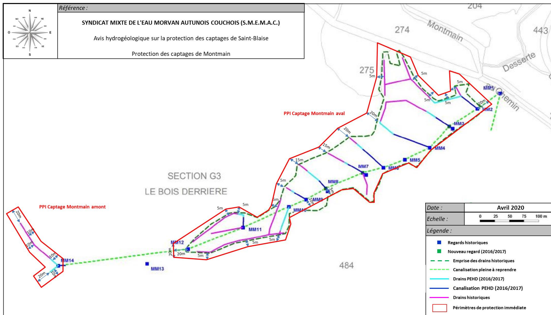
Figure 7 : délimitation des périmètres de protection immédiate des captages amont et aval de Montmain
