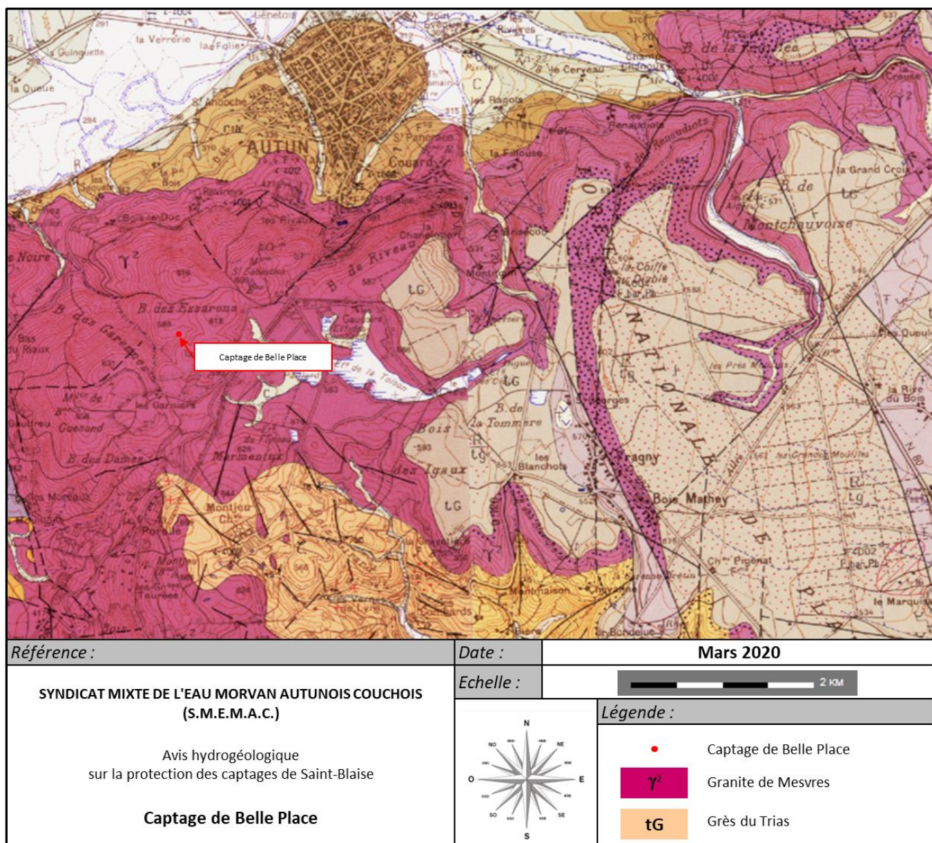
Figure 4 : localisation du captage de Belle Place sur extrait de carte géologique au 1/50 000 e , feuille d'Autun
