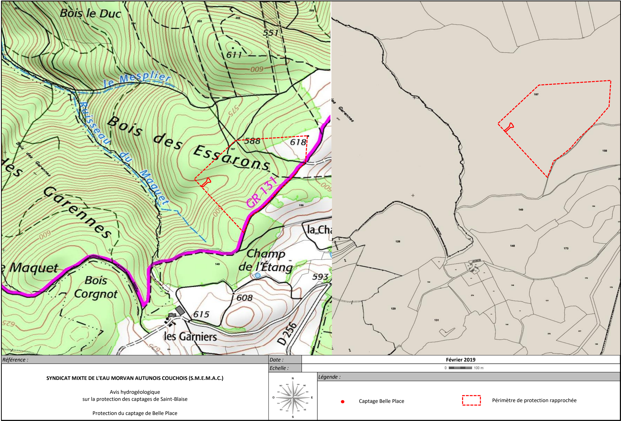
Figure 10 : délimitation du périmètre de protection rapprochée du captage de Belle-Place sur fonds IGN et cadastral
