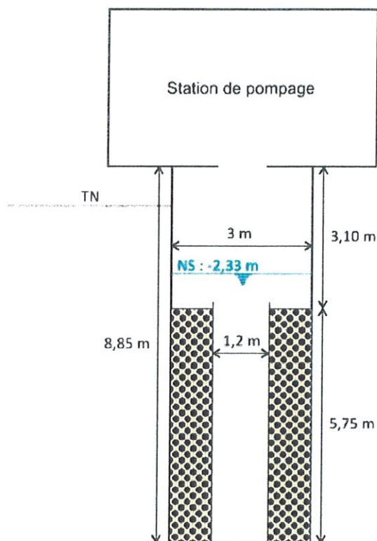
Figure 6 : Coupe schématique du puits
