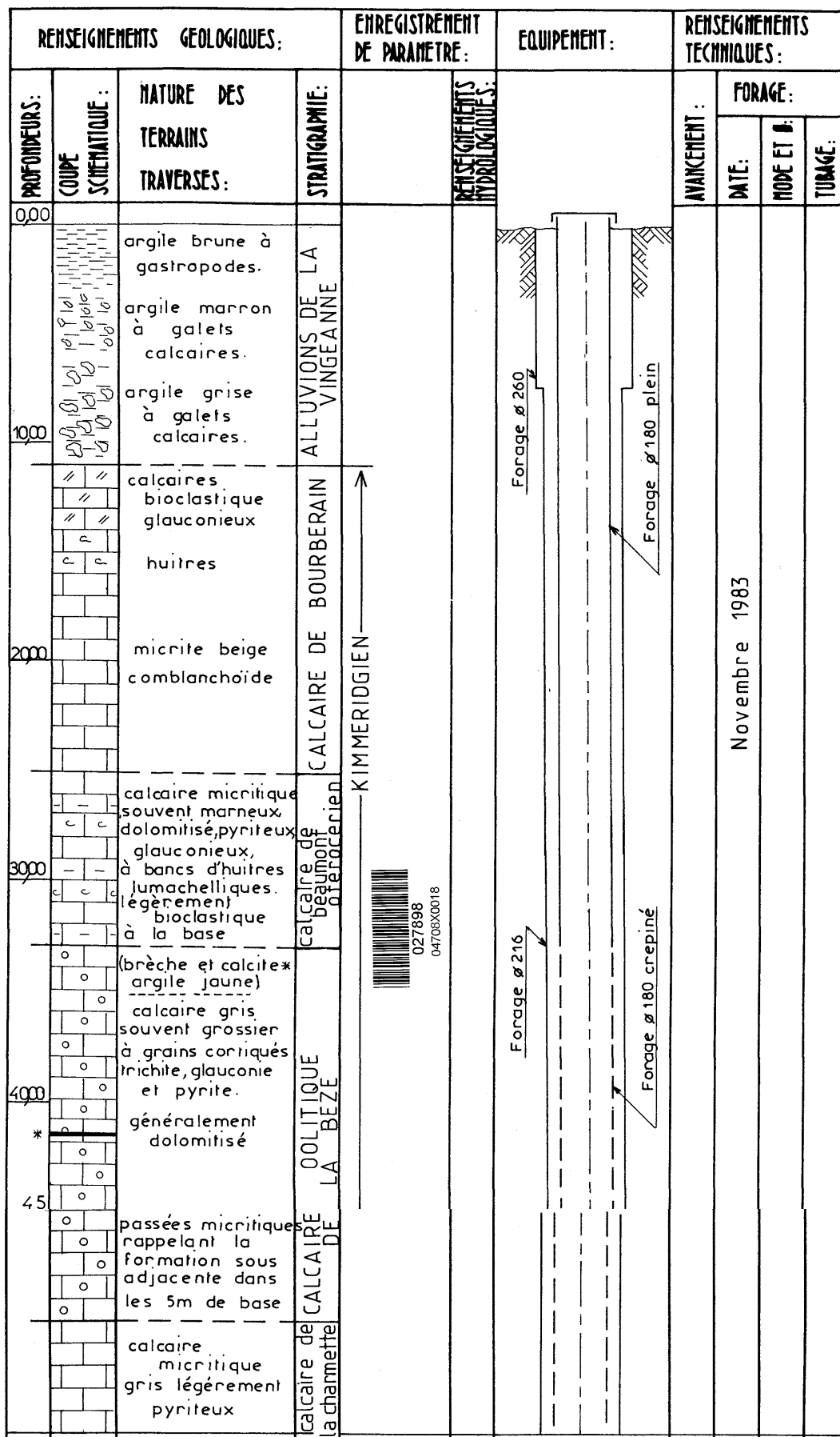
Figure 3 : Coupe géologique et technique du puits d'Oisilly
