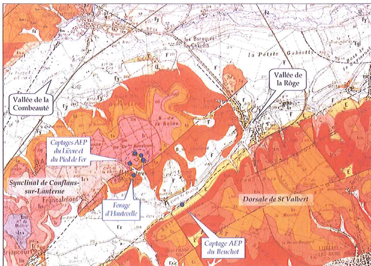
Extrait de la carte géologique B.R.G.M. 1/50 000 e de Luxeuil-les-Bains
